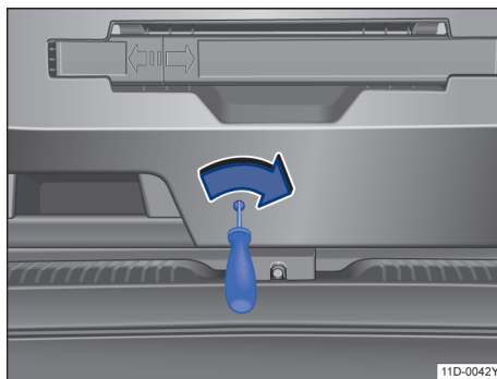
图 56 行李厢应急解锁
