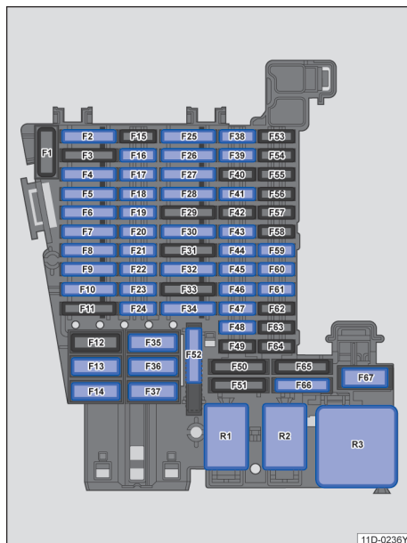
图 142 保险丝位置示意图
