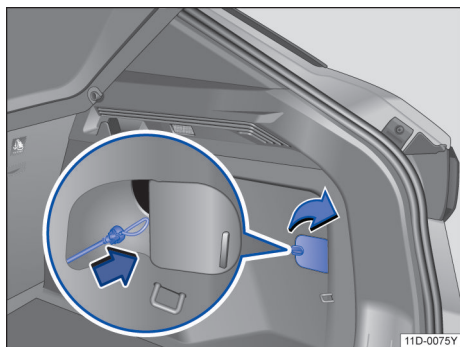
图 136 行李厢内的交流充电插头应急解锁拉索
