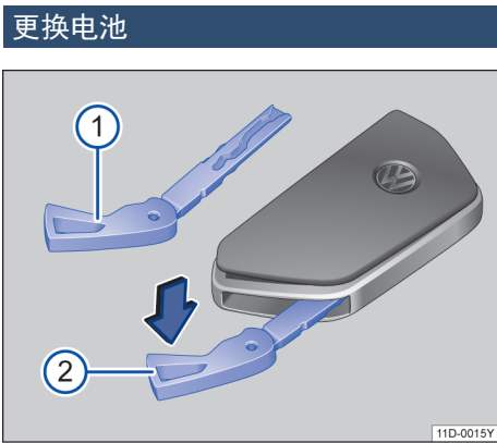
图 41 汽车钥匙：打开电池盒盖板
