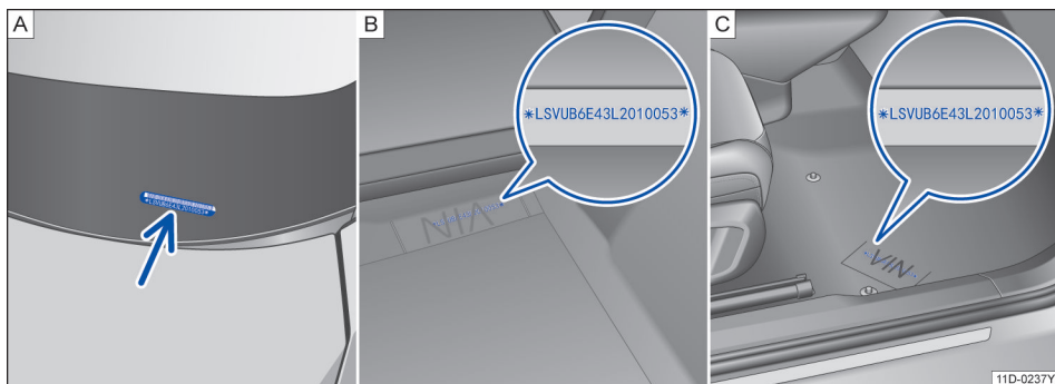
图 161 A. 车辆识别代号 B. 第二排座椅后侧的车辆识别代号钢印位置 或 C. 副驾驶座椅下方的车辆识别代号钢印位置
