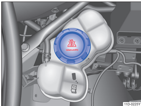
图 155 冷却液补偿容器盖
