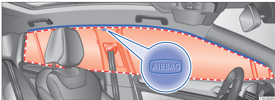
图 32 在汽车左侧：头部安全气囊的安装位置和膨胀范围
