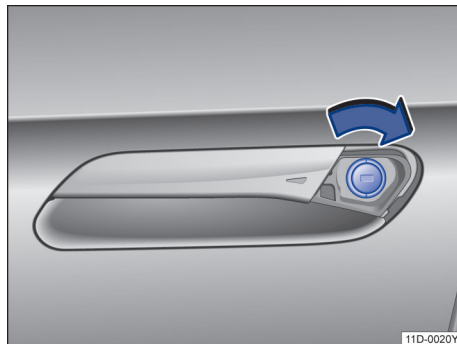
图 47 驾驶员车门紧急锁止
