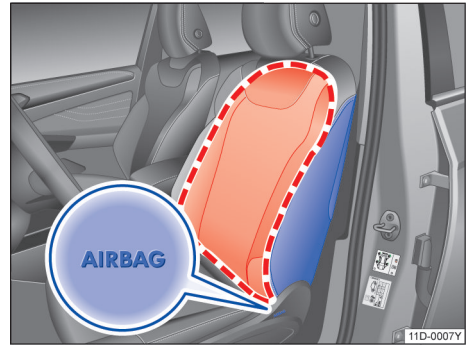
图 31 前排座椅侧面：侧面安全气囊的安装位置和膨胀范围
