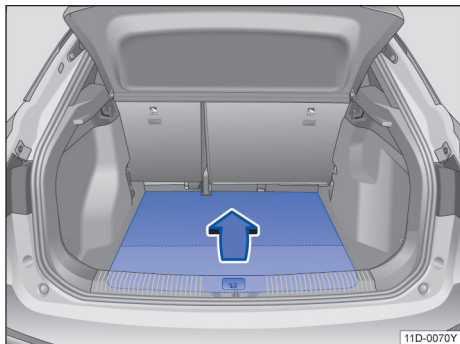
图 126 行李厢内：抬起行李厢地板
