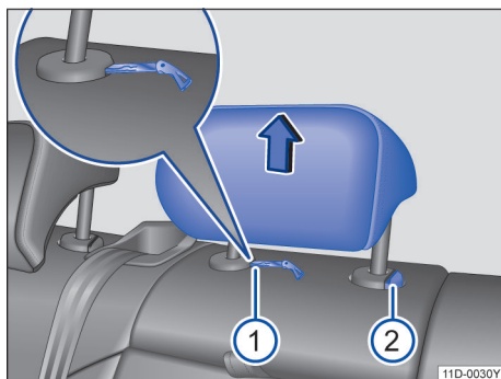
图 68 拆卸和安装后排头枕
