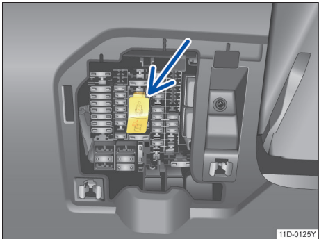
图 143 救援用保险丝
