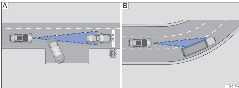
图 99 [A]. 正在转弯和静止的车辆 [B]. 弯道行驶
