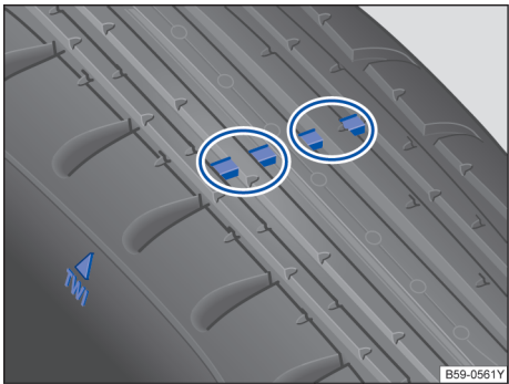
图 157 轮胎花纹磨损标记
