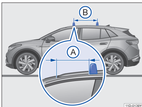
图 128 配备车顶行李架基架的汽车：行李架杆的固定点
