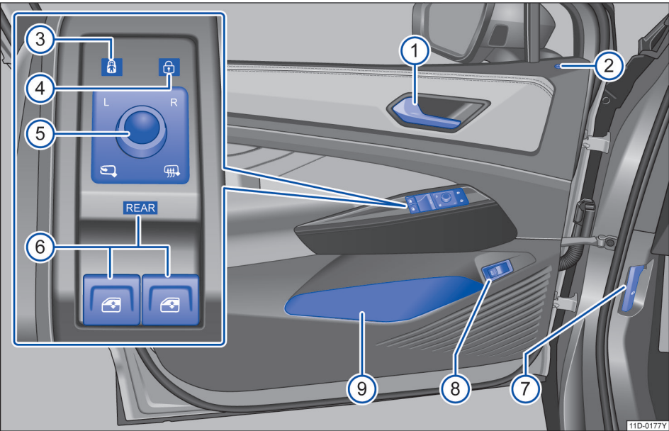
图 3 驾驶员侧车门内的操作元件概览
