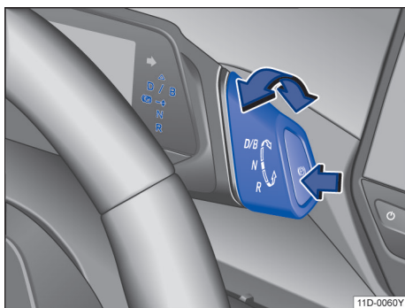
图 93 带电子驻车制动器按钮的行驶挡开关（箭头）
