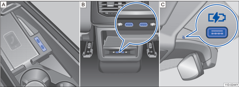
图 123 A. 前排位于储物盒内的 Type-C 插口 B. 后排位于出风口下方 Type-C 插口 C. 车顶 Type-C
